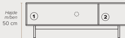
Højde m/ben 50 cm H2HA 2 sektioner Med flip-dør + dør til højre 2 rum 144x30x33 cm
